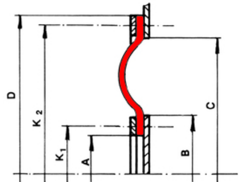
Anmerkung | Typ 35 - Weichstoff-Kompensator | Maßskizze
